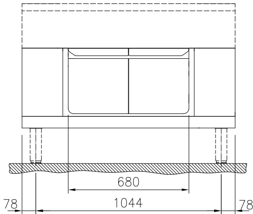
Zij aanzicht
